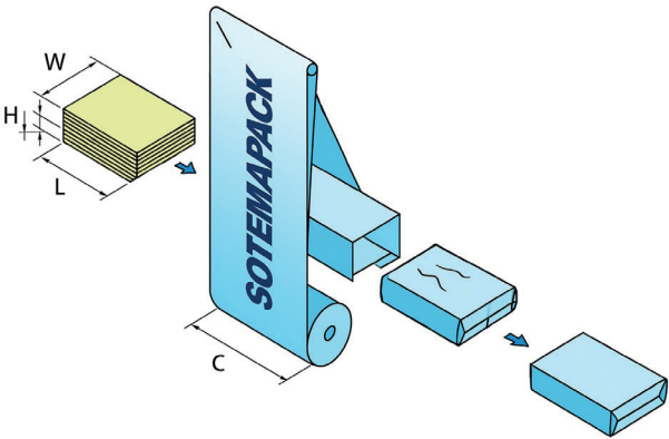
Configurazione con bobina monopiega Configuration by ½ tube film reel
