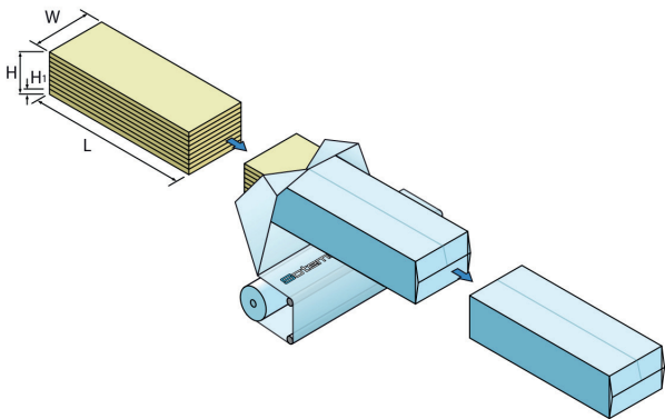
Configurazione con bobina piana aperta Configuration with spool flat leaf
